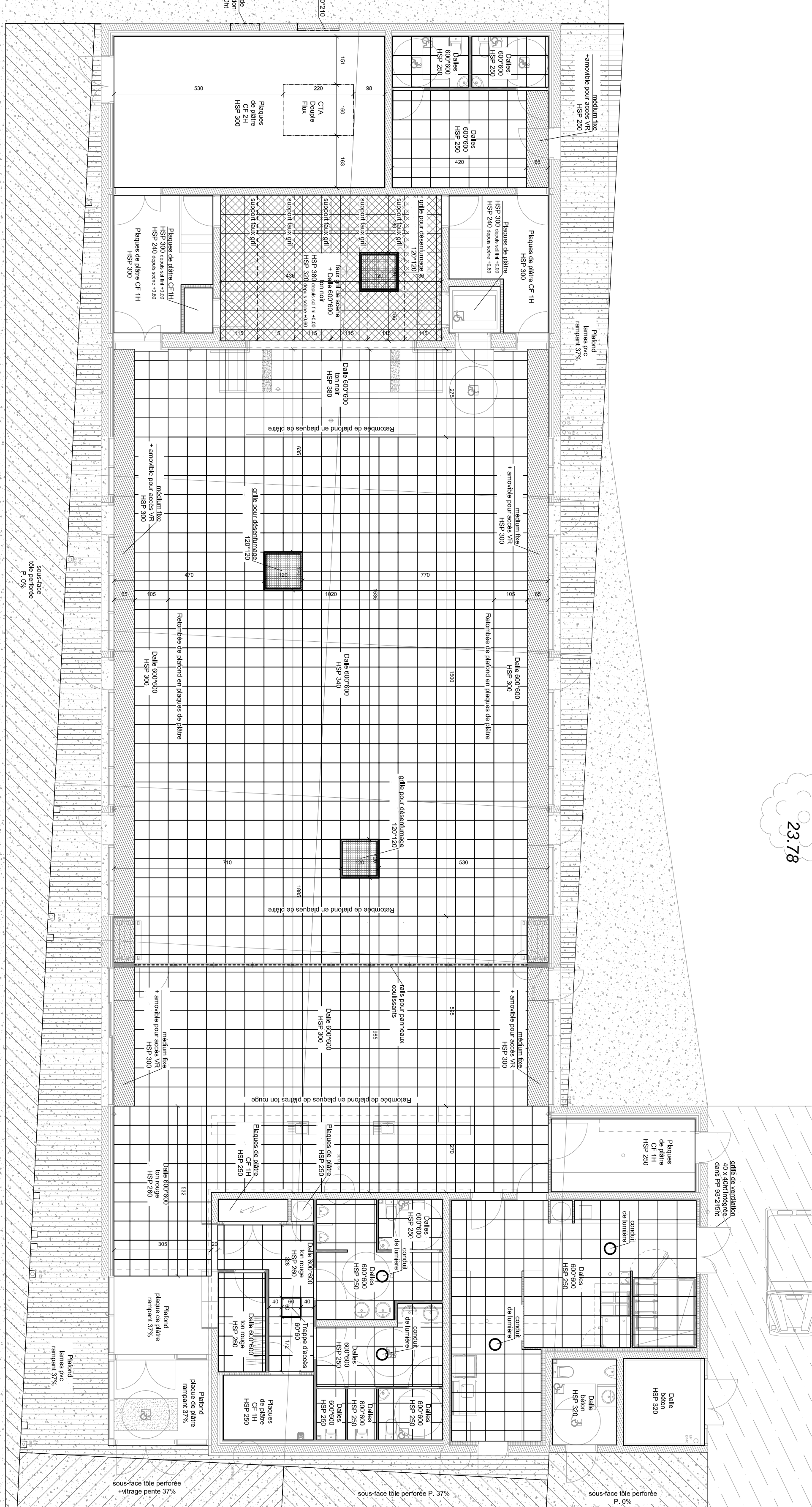
PLAN PLAFOND - ECH 1/100°
