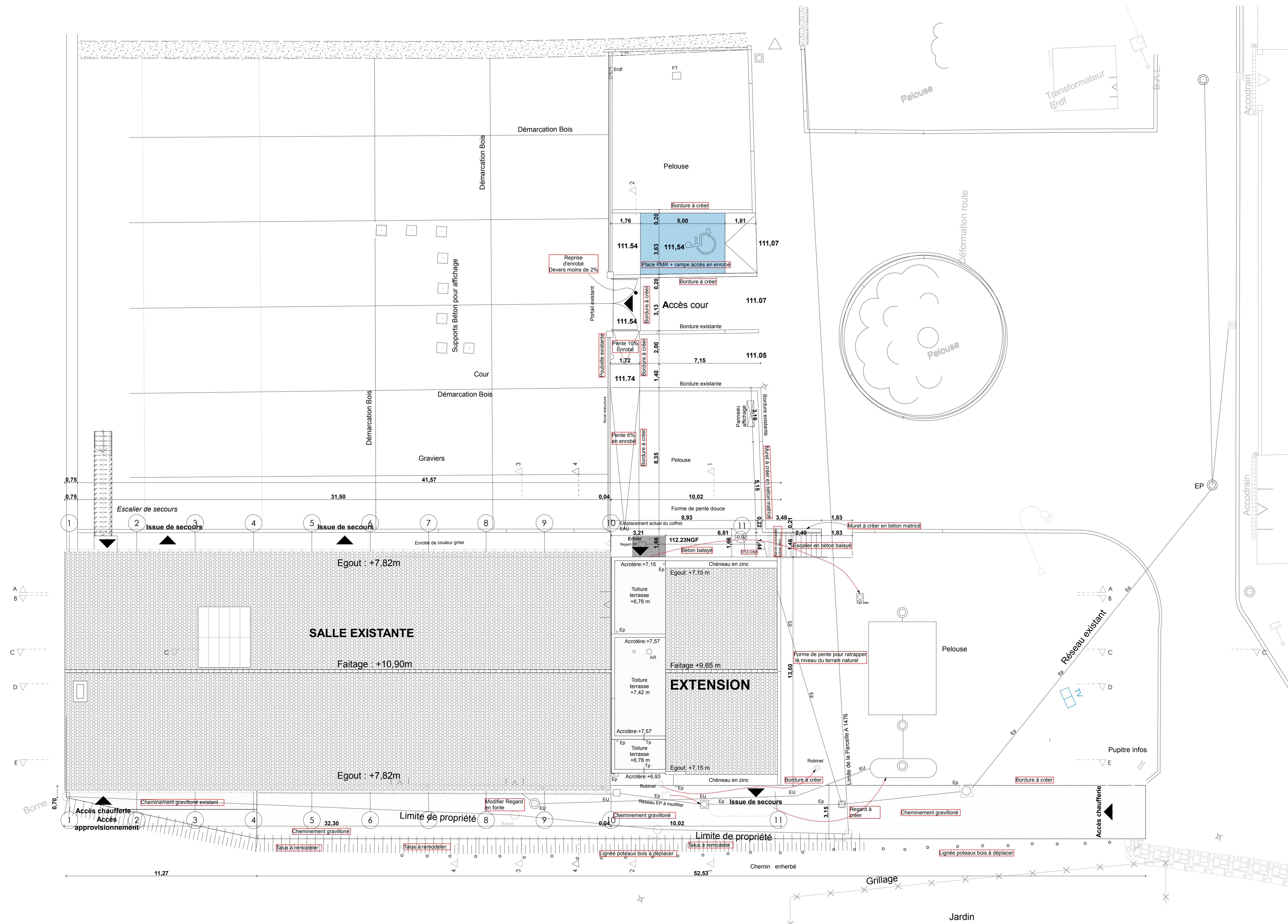
PLAN MASSE
