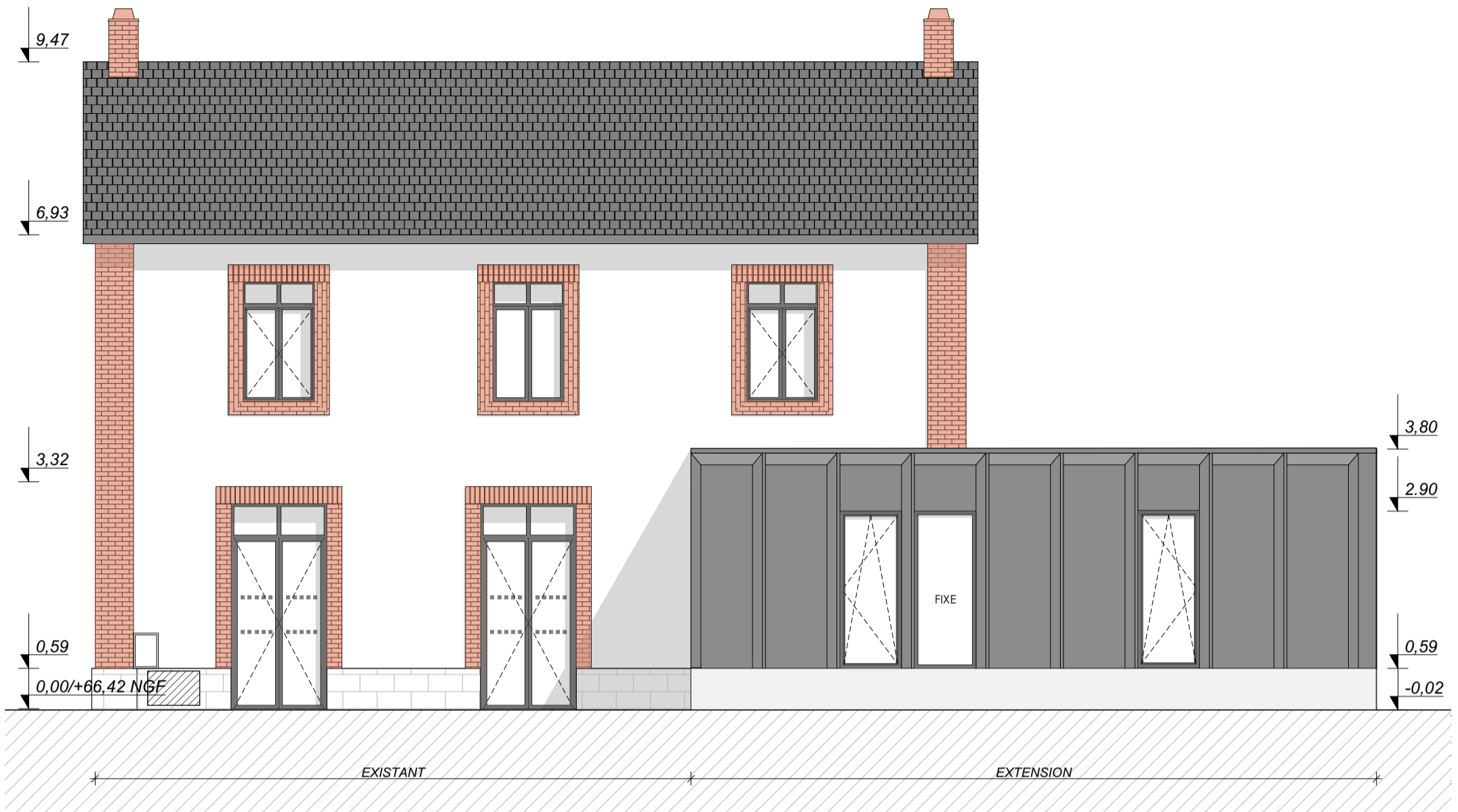
_Façade Nord-Ouest projetée 1/75
