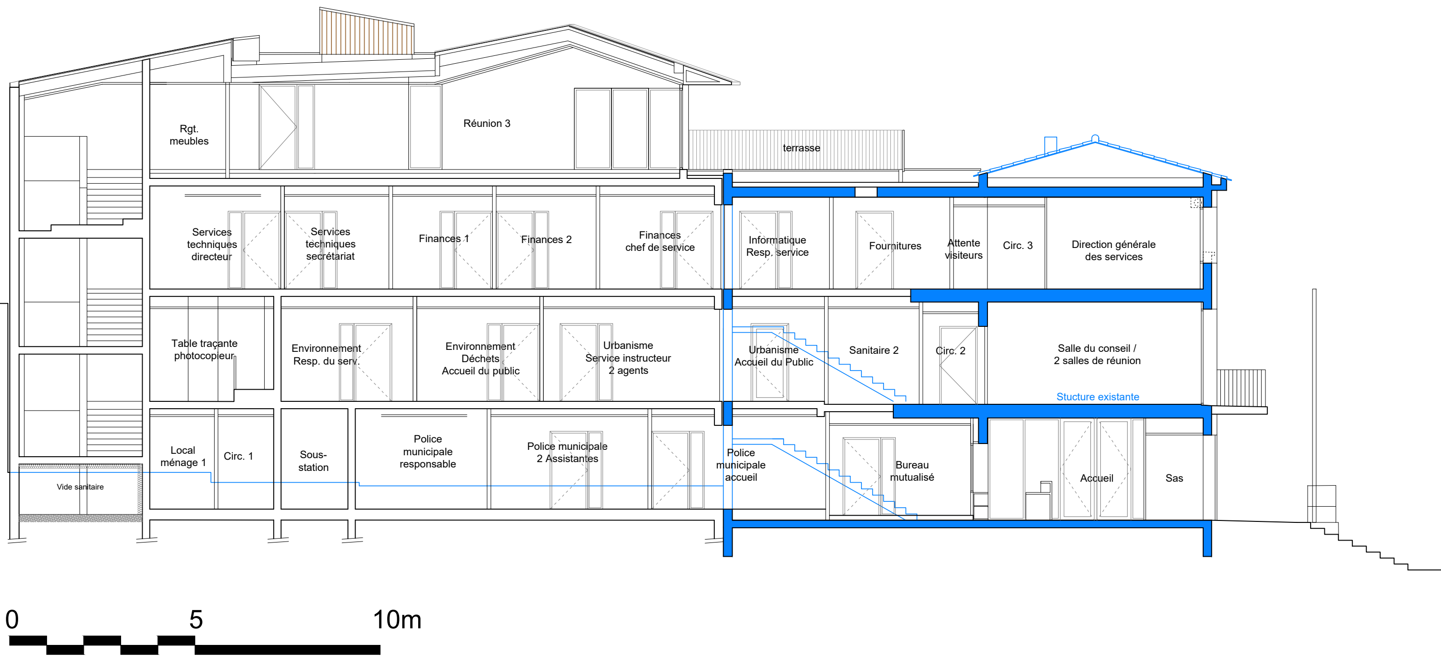
Coupe
